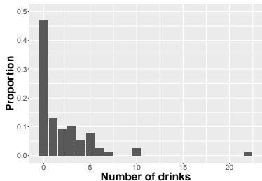
(a) Actual distribution
